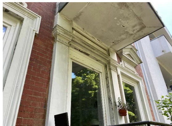
Einbausituation Balkontür
