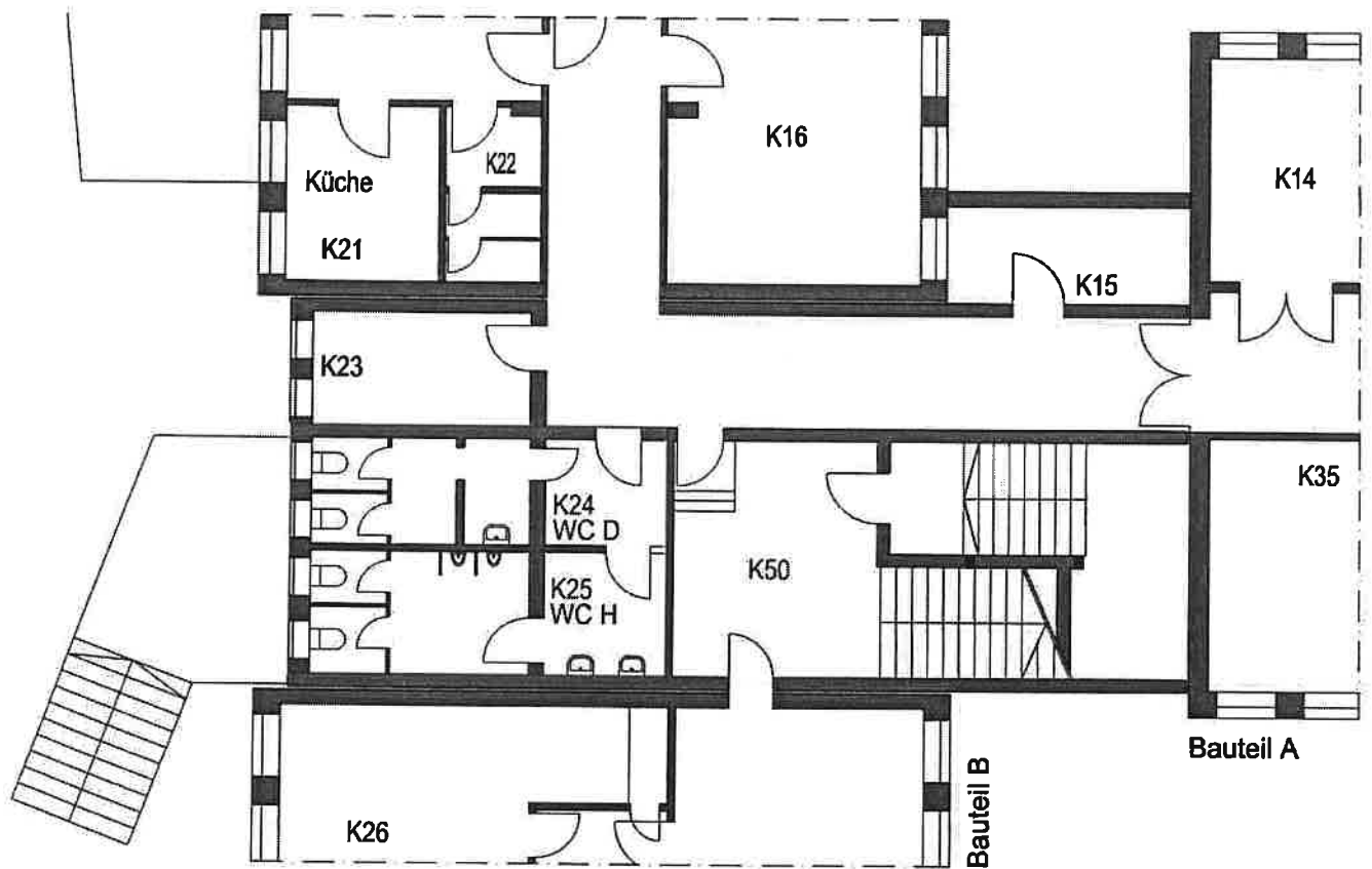
Bauteil B Kellergeschoss
