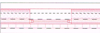
02 Dachflächenfenster Nord-Ost
